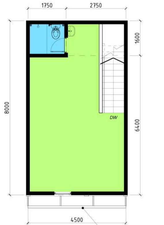
DENAH LT.2 SKALA 1 : 100
