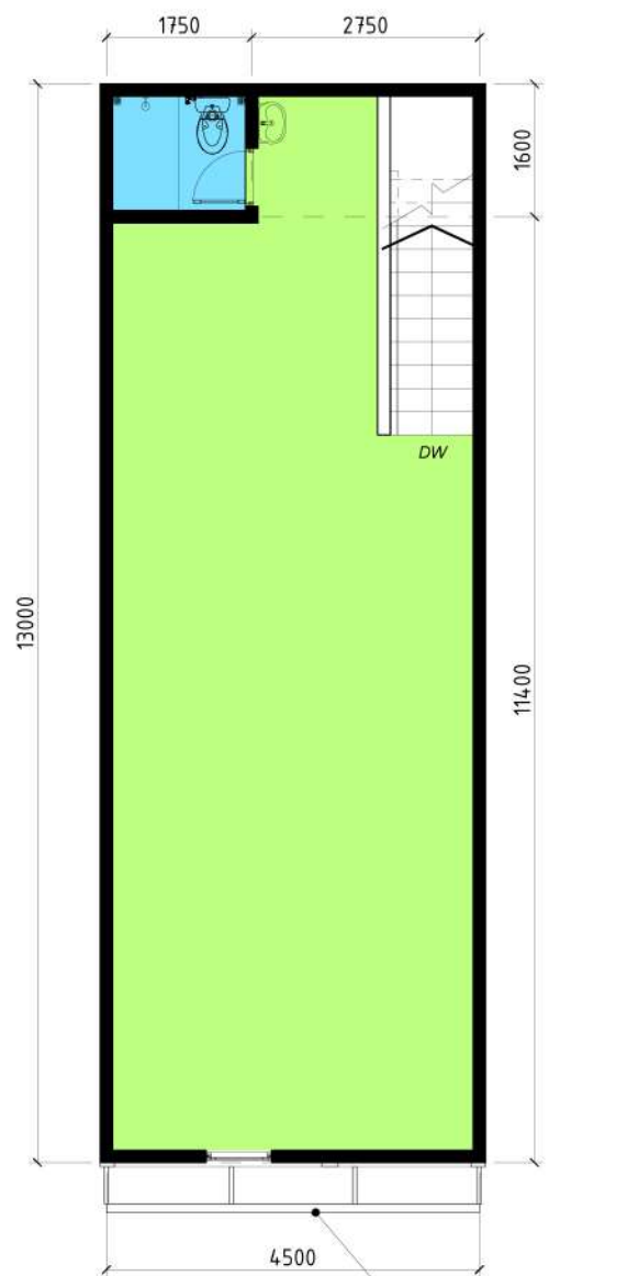
DENAH LT.2 SKALA 1 : 100
