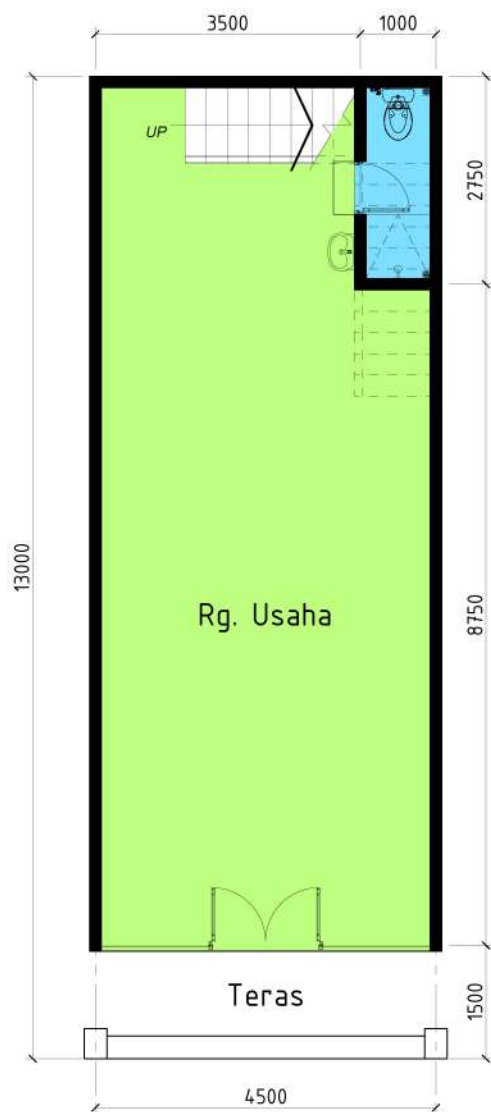
DENAH LT.1 SKALA 1 : 100
